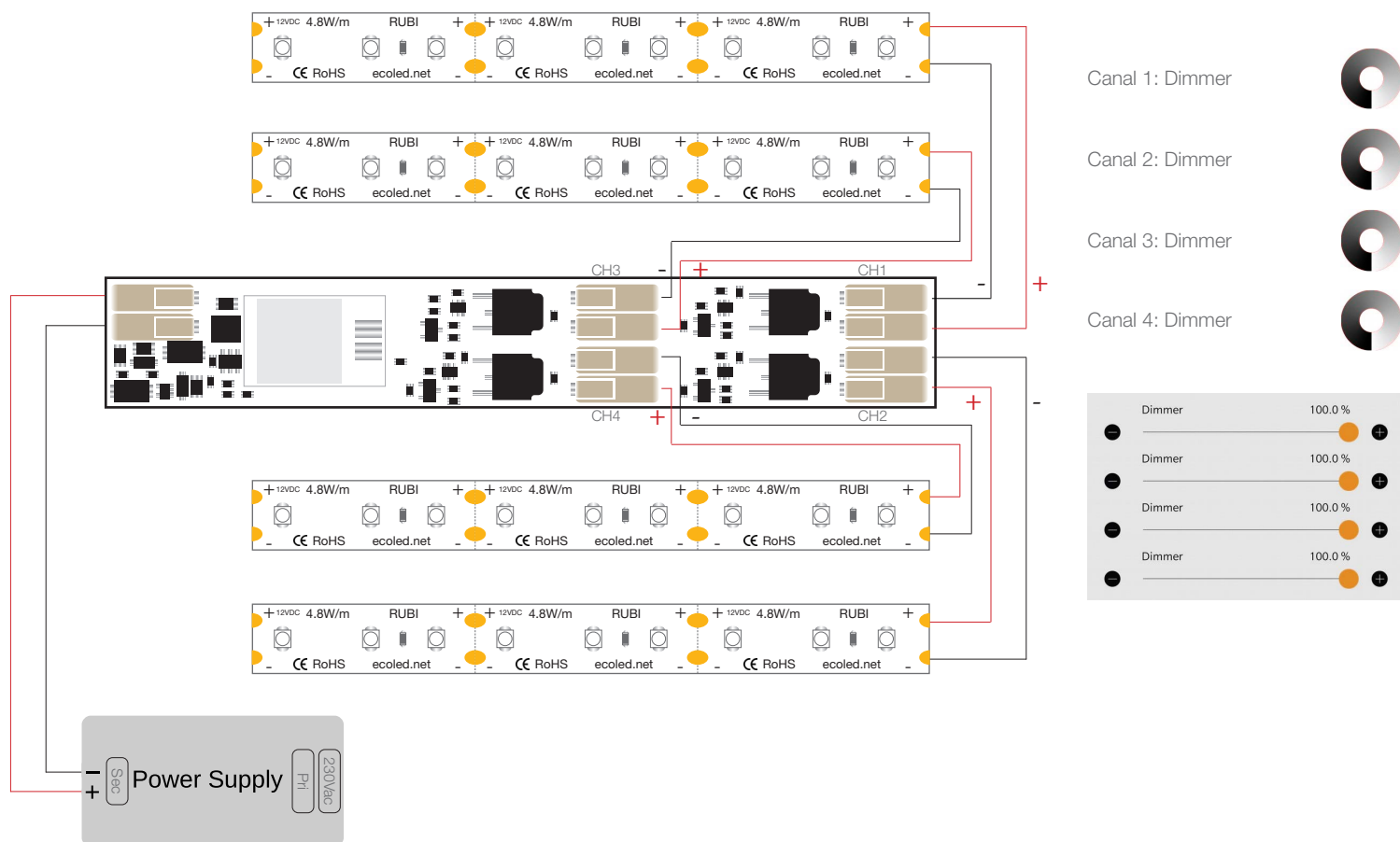
Diagrama con 4 canales separados
